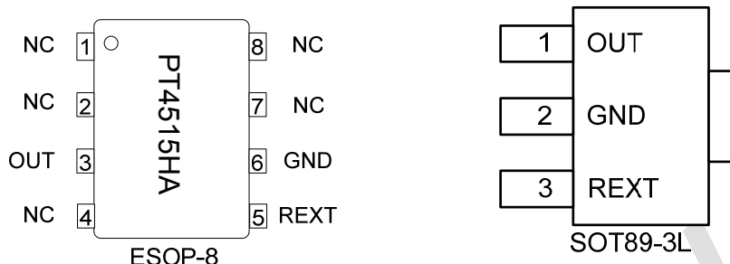
图 2. PT4515HA 管脚定义图
