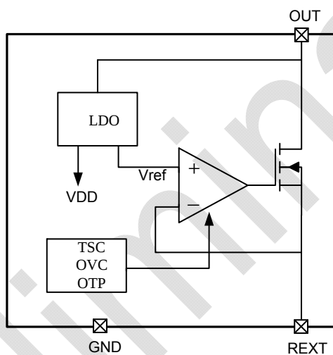
图 3. PT4515HA 内部模块简化图
