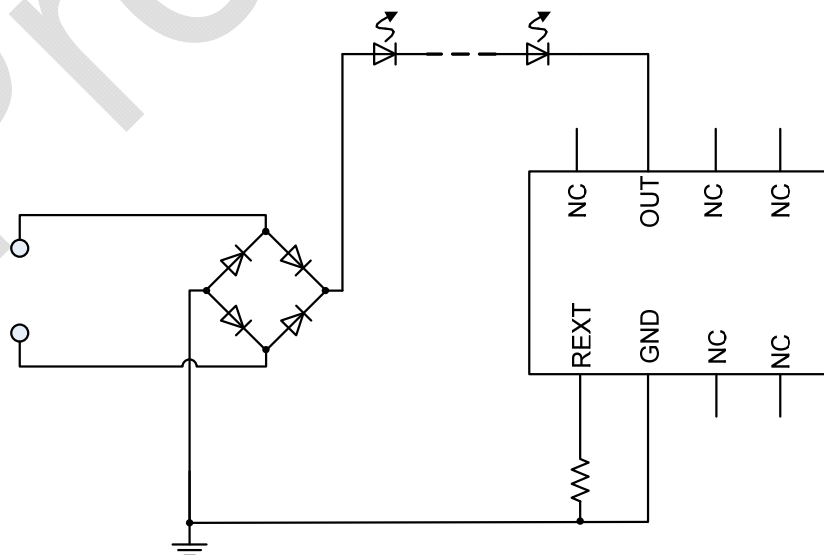
图 1. PT4515HA 典型应用电路图
