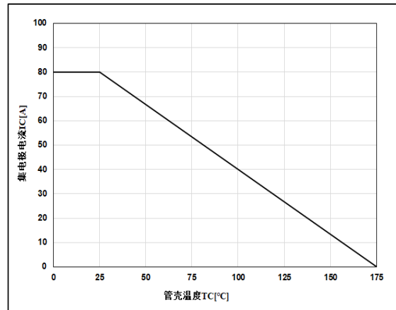
图 16 集电极电流温度特性 ( T_J \leq 175^\circ C )
