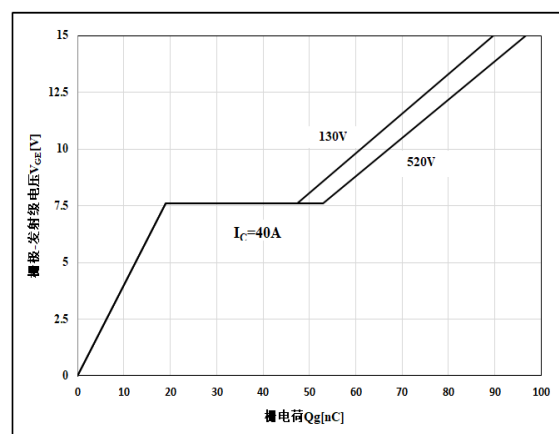
图 18 栅电荷特性
