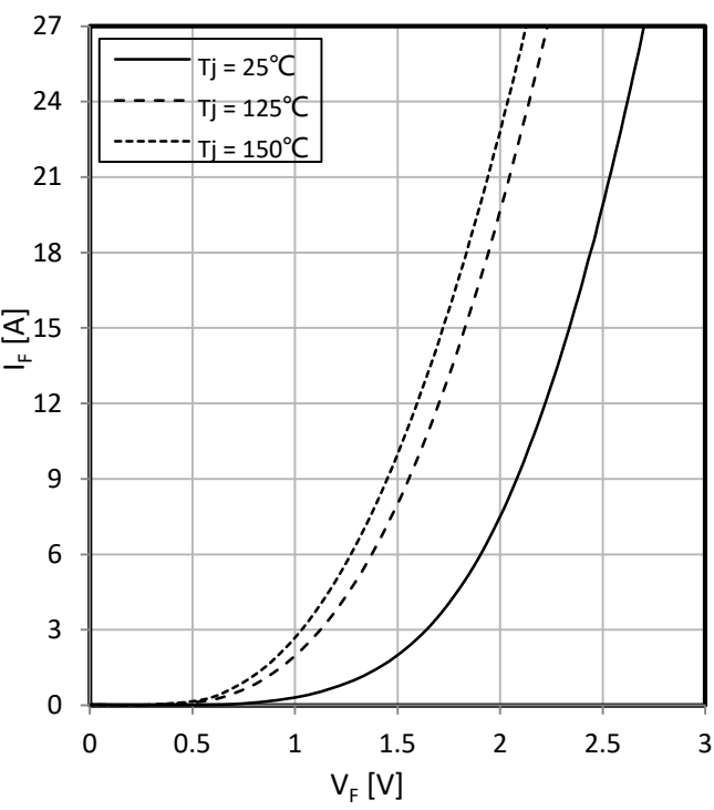
正向偏压特性 二极管，制动-斩波器（典型） Forward characteristic of Diode, Barke-Chopper (typical) I_F = f(V_F)
