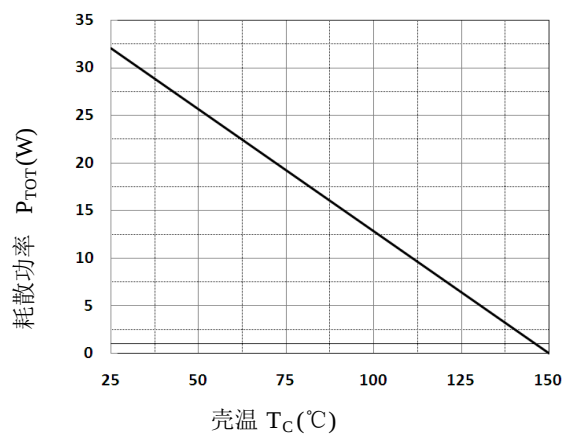
图 15. 耗散功率—壳温 T_C 特性
