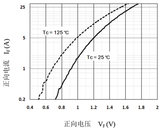
图 17. 二极管正向压降特性
