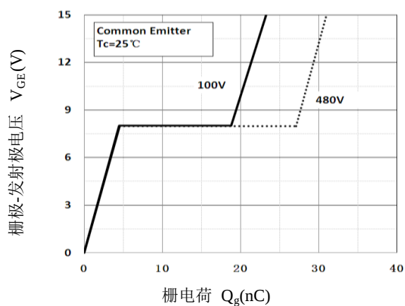
图 16. 栅电荷特性
