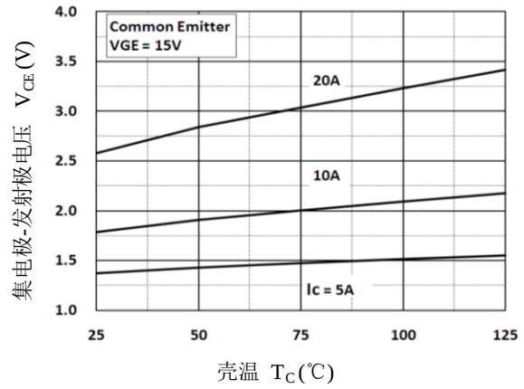
图 4. 饱和压降—温度特性
