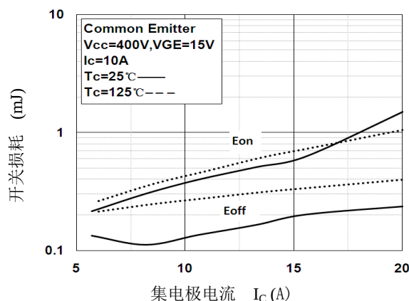
图 8. 开关损耗— I_C 特性
