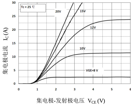
图 1. 输出特性
