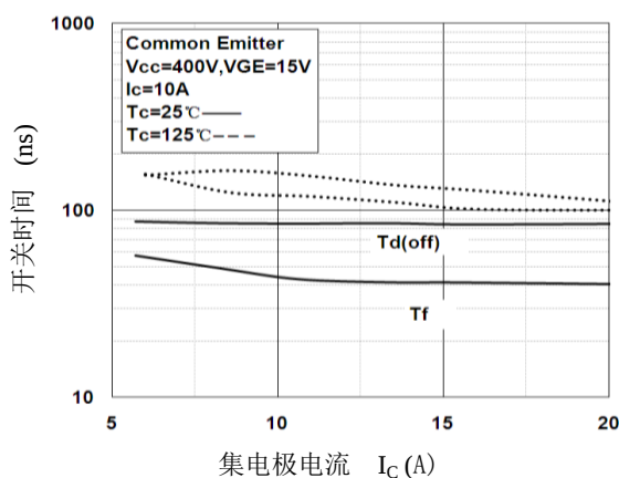
图 9. 开关时间— I_C 特性
