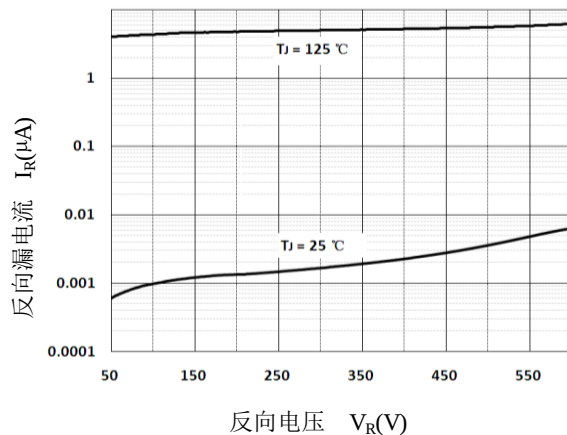
图 18. 二极管反向漏电特性
