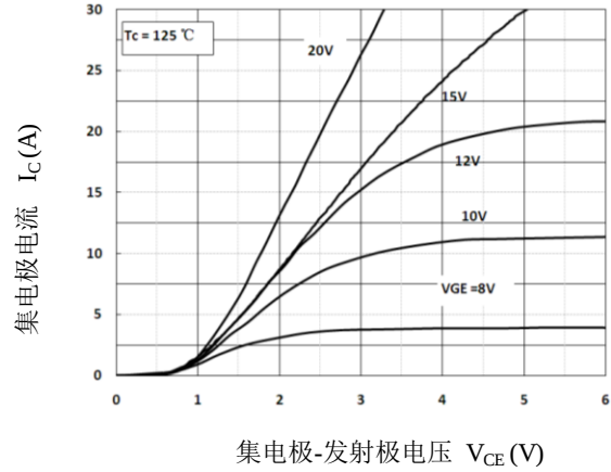
图 2. 输出特性
