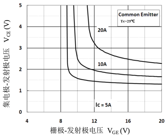
图 5. 饱和压降— V_{GE} 特性
