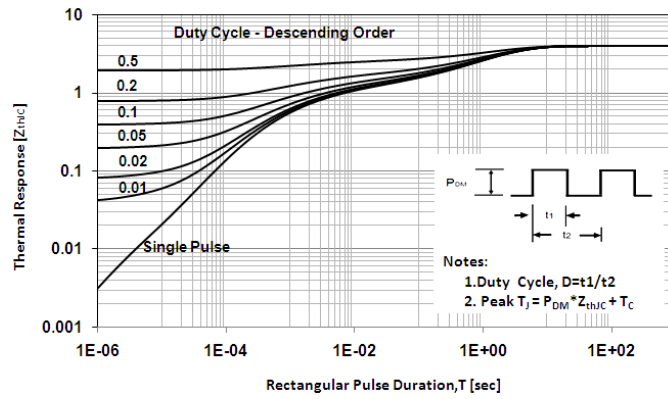
图 19. IGBT 瞬态热阻特性
