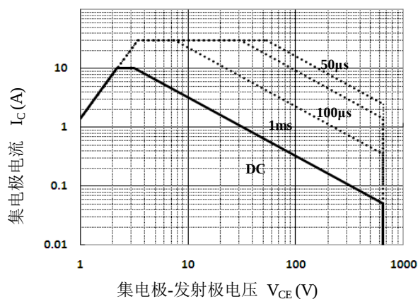
图 14. 安全工作区
