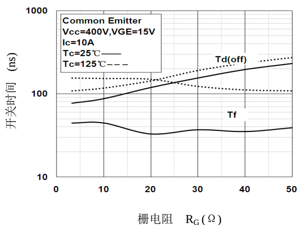
图 12. 关断时间— R_G 特性
