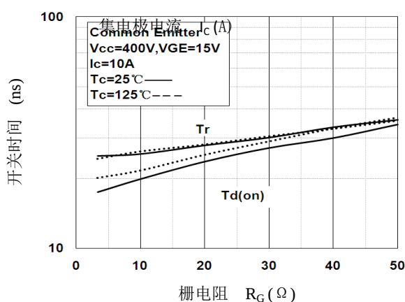
图 10. 开关时间— R_G 特性
