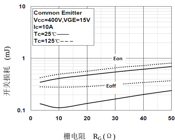
图 11. 开关损耗— R_G 特性
