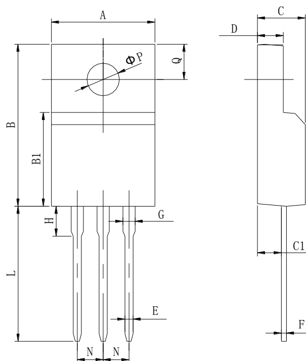
外形图: CRG20T60A93L (TO-220F)
