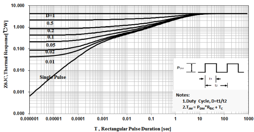
图 23 瞬态热阻特性-220F
