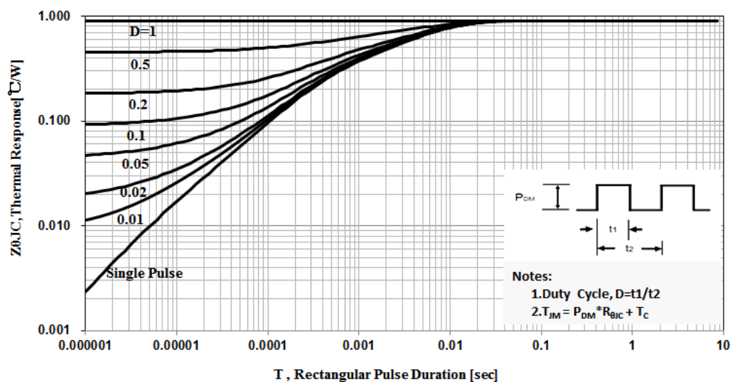
图 22 瞬态热阻特性-220
