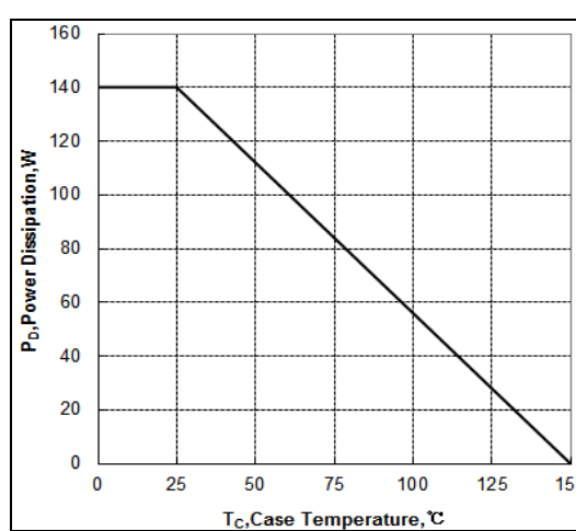
图 18 耗散功率-壳温 T_c 特性 (220F)
