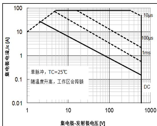
图 20 正向安全工作区-220
