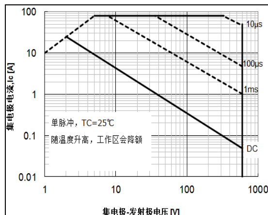
图 21 正向安全工作区-220F
