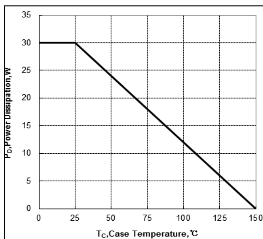
图 17 耗散功率-壳温 T_c 特性 (220AB)
