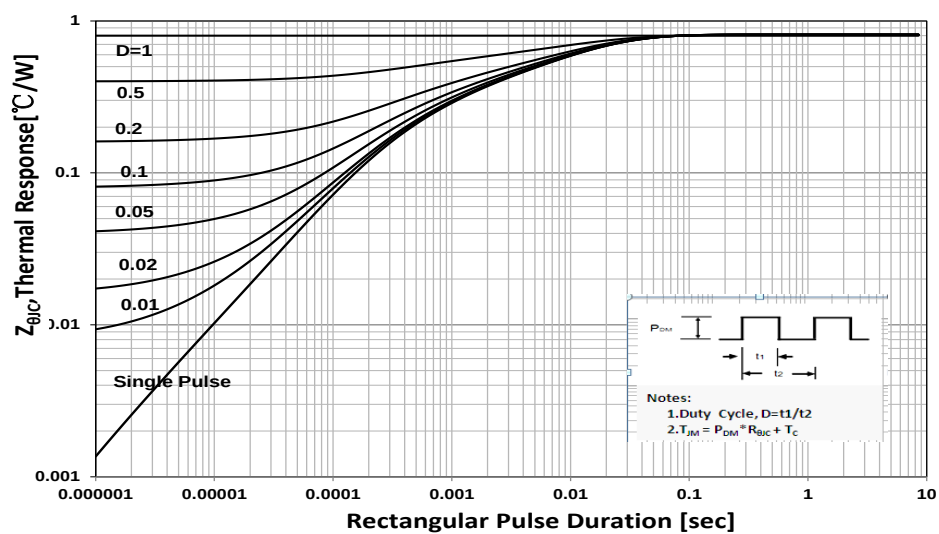
图 19 瞬态热阻特性
