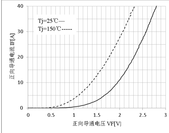
图 17 二极管正向特性
