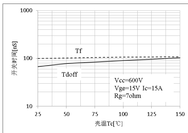
图 12 关断温度特性
