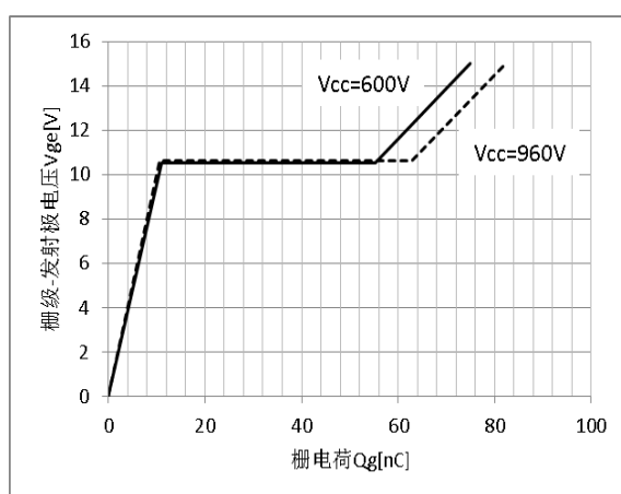
图 6 栅电荷特性
