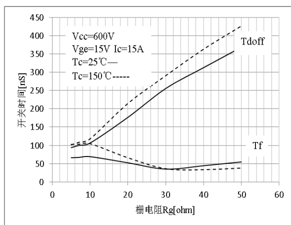
图 9 关断-栅电阻特性曲线
