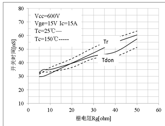
图 8 开通-栅电阻特性曲线
