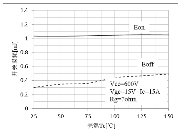
图 10 开关损耗温度特性
