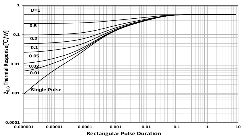
图 19 瞬态热阻特性
