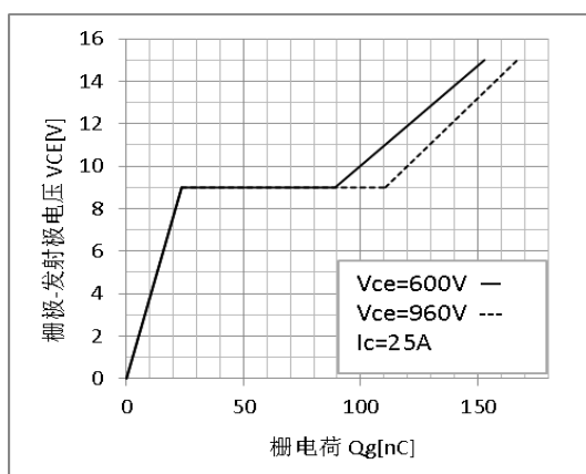
图 6 栅电荷特性
