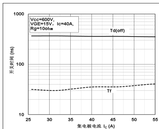
图 14 关断与电流特性
