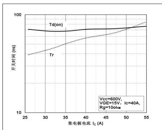
图 15 开通与电流特性
