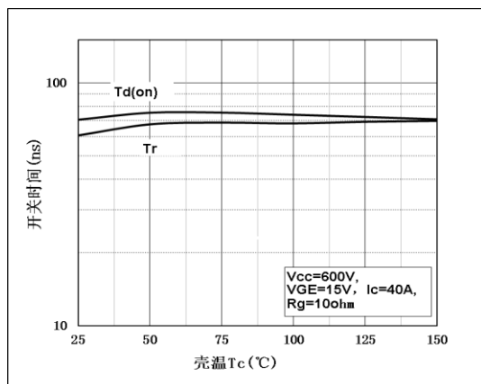
图 11 开通温度特性
