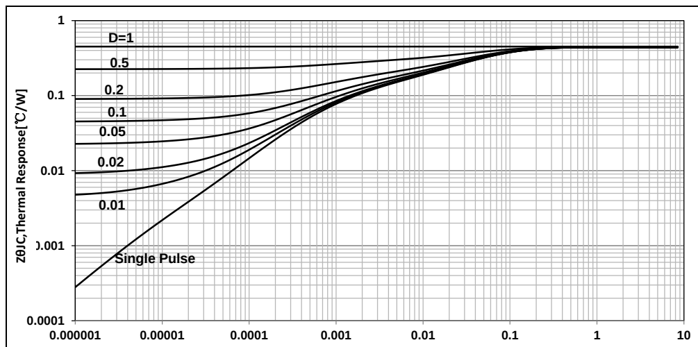
图 19 瞬态热阻特性
