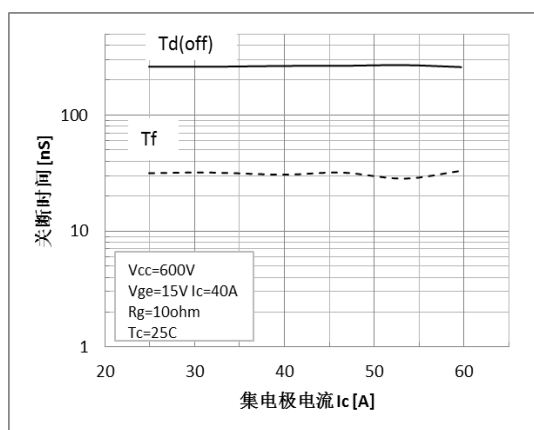
图 15 关断与电流特性
