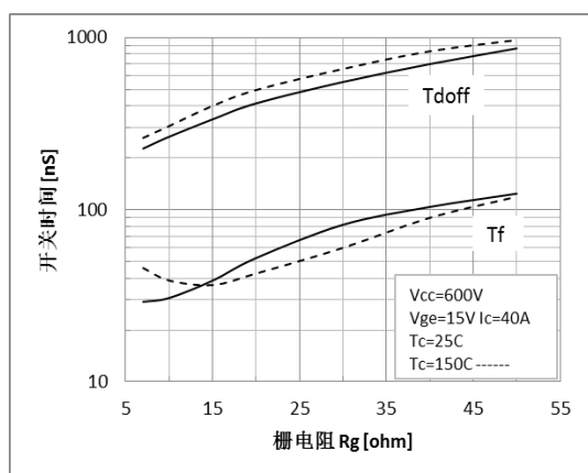
图 9 关断-栅电阻特性曲线
