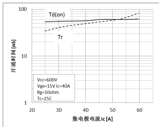
图 14 开通与电流特性
