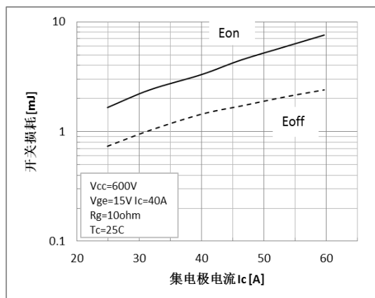
图 13 开关损耗与电流特性
