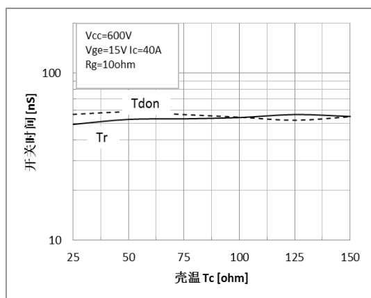
图 11 开通温度特性
