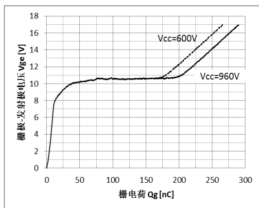
图 6 栅电荷特性
