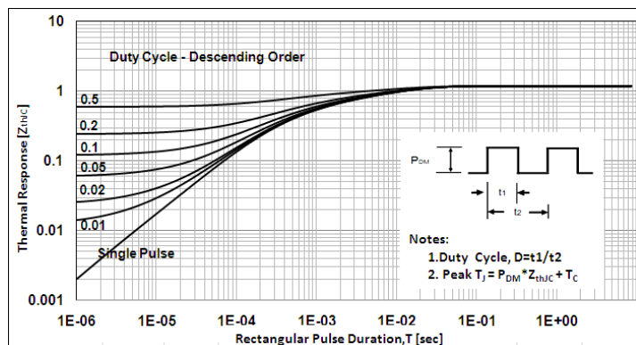
图 19. IGBT 瞬态热阻特性
