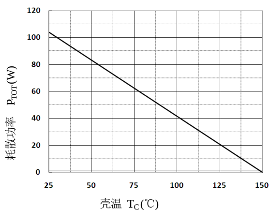
图 15. 耗散功率—壳温 T_C 特性
