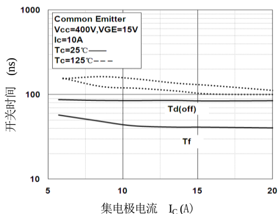
图 9. 开关时间— I_C 特性
