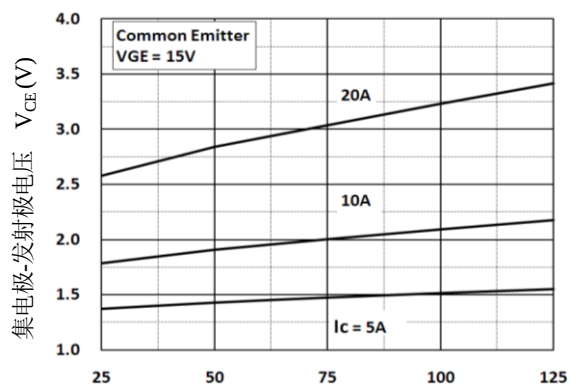
壳温 T_c (°C)
