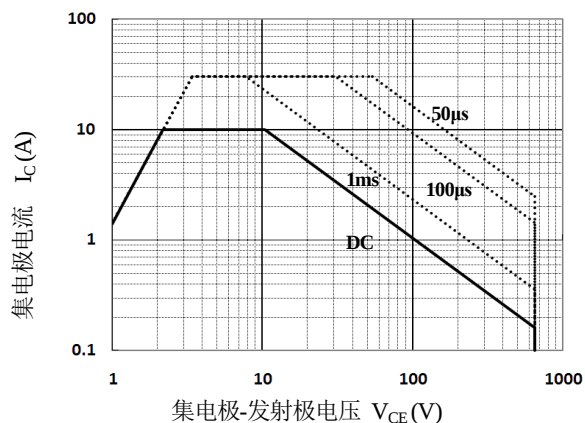
图 14. 安全工作区
