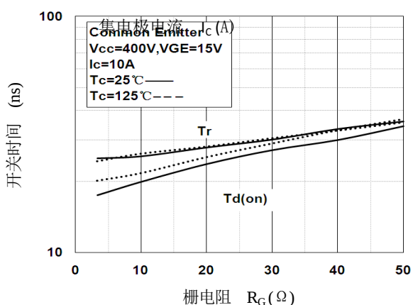
图 10. 开关时间— R_G 特性
