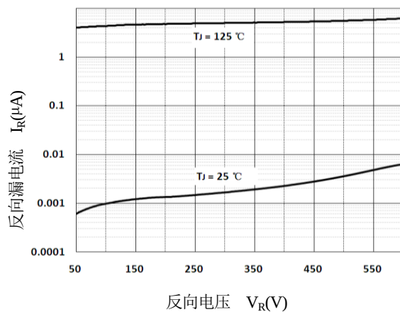
图 18. 二极管反向漏电特性
