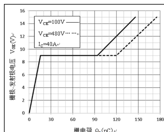
图 18 栅电荷特性
