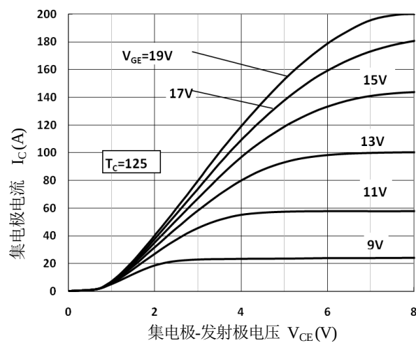
图 2. 输出特性
