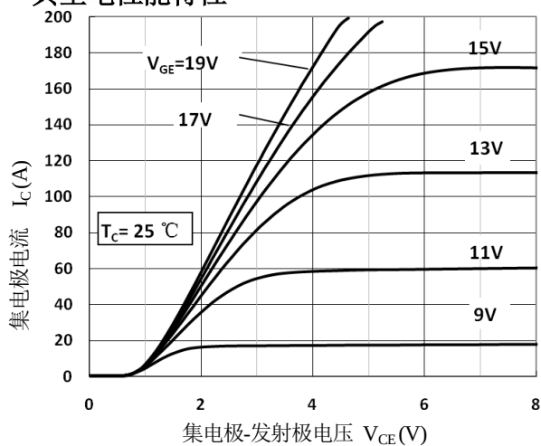
图 1. 输出特性
