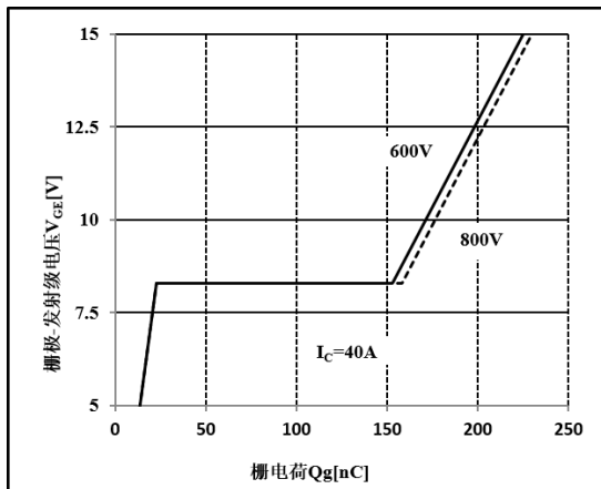
图 18 栅电荷特性
