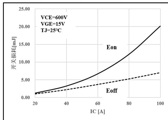
图 12 开关损耗的电流特性
