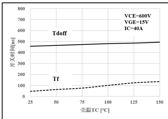
图 11 关断温度特性
