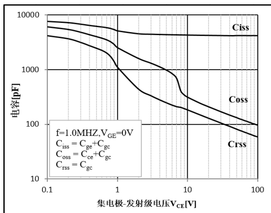
图 5 电容特性
