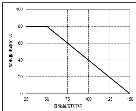
图 16 集电极电流温度特性
