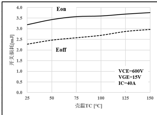
图 9 开关损耗温度特性
