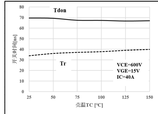
图 10 开通的温度特性
