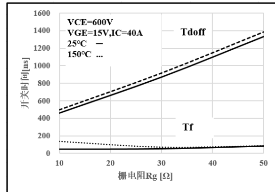
图 8 关断-栅电阻特性曲线
