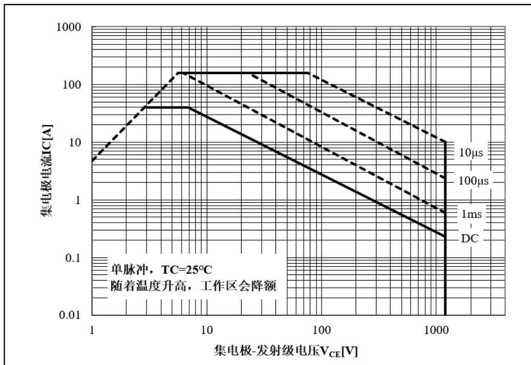
图 19 正向安全工作区
