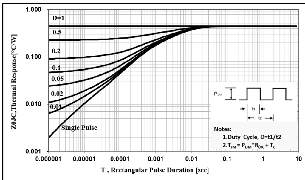
图 20 瞬态热阻特性
