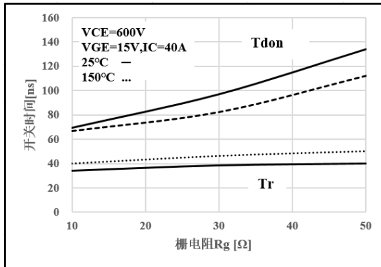
图 7 开通-栅电阻特性曲线
