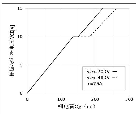
图 18 栅电荷特性
