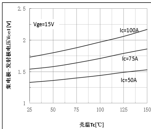
图 4 饱和压降温度特性
