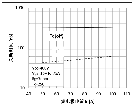
图 14 关断的电流特性
