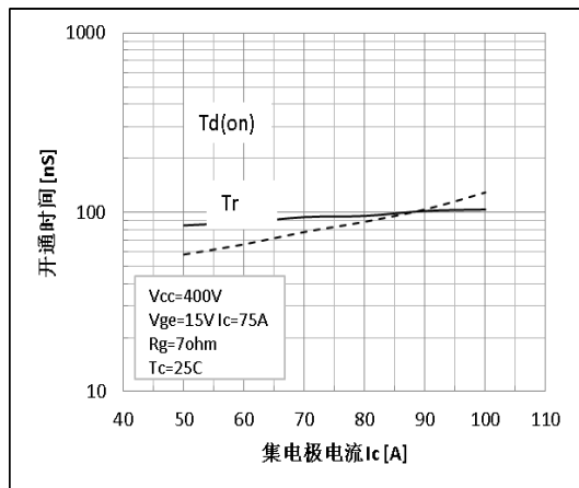
图 13 开通的电流特性
