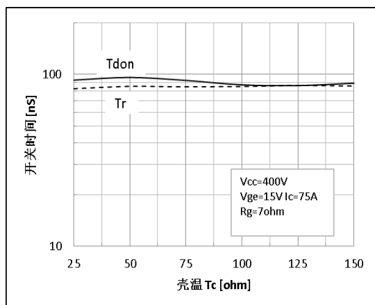
图 11 开通的温度特性
