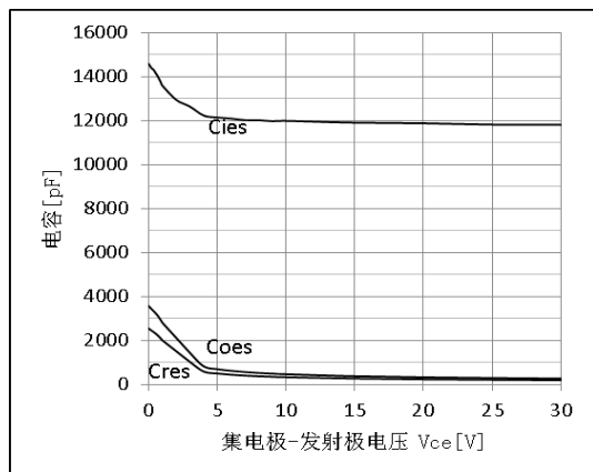
图 5 电容特性
