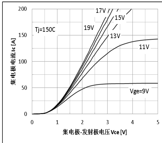
图 2 输出特性曲线
