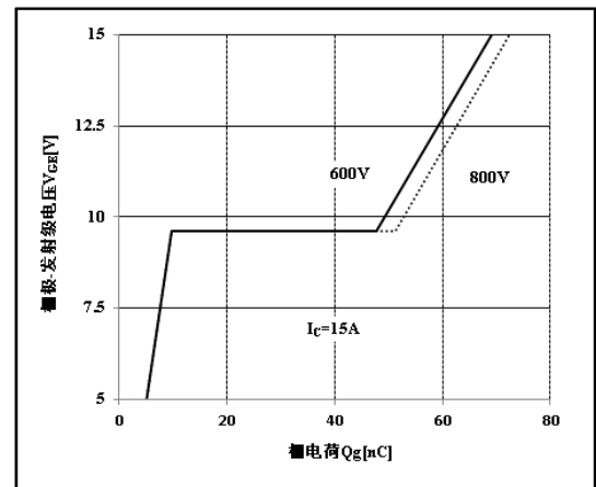
图 18 栅电荷特性
