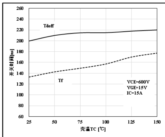
图 11 关断温度特性
