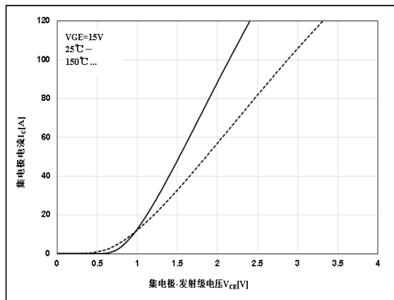
图 3 饱和和压降特性
