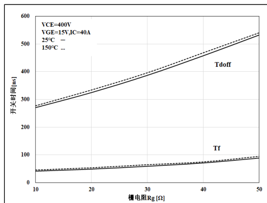
图 8 关断-栅电阻特性曲线
