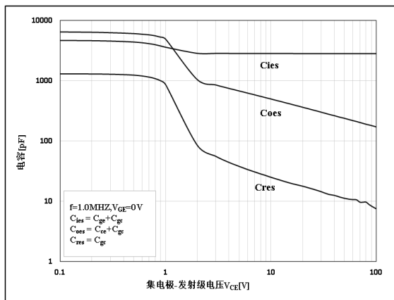
图 5 电容特性
