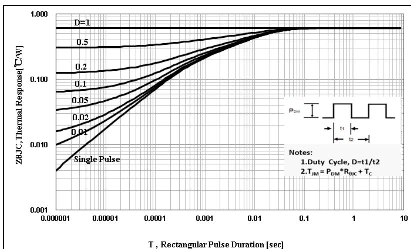
图 20 瞬态热阻特性
