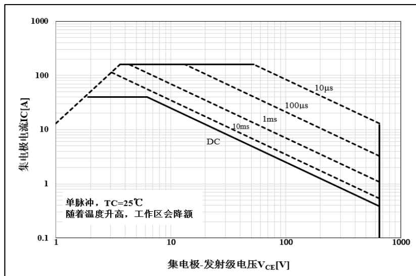
图 19 正向安全工作区
