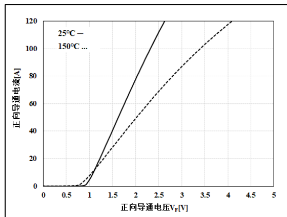
图 15 二极管正向特性
