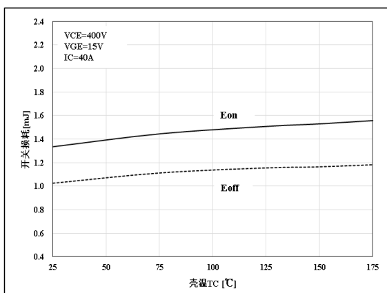
图 9 开关损耗温度特性
