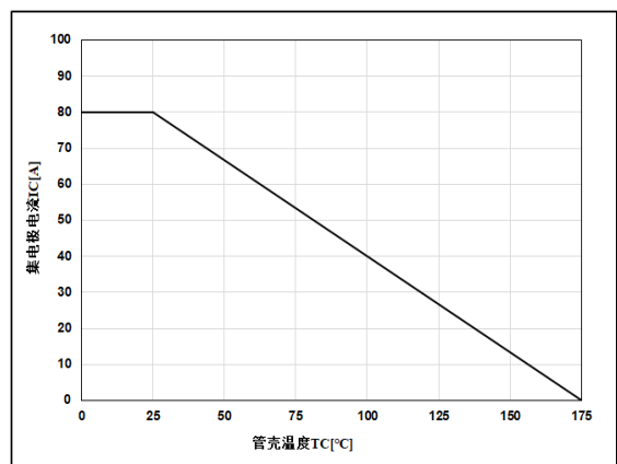
图 16 集电极电流温度特性 ( T_j \leq 175^\circ\text{C} )
