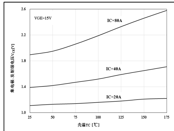
图 4 饱和和压降温度特性
