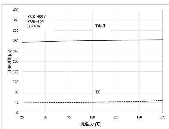
图 11 关断温度特性
