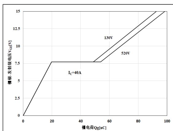
图 18 栅电荷特性
