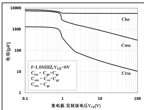
图 5 电容特性
