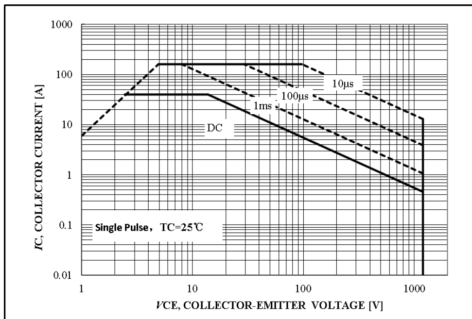
图 19 正向安全工作区
