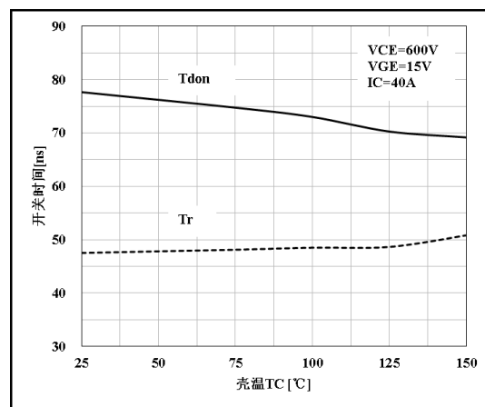
图 10 开通温度特性
