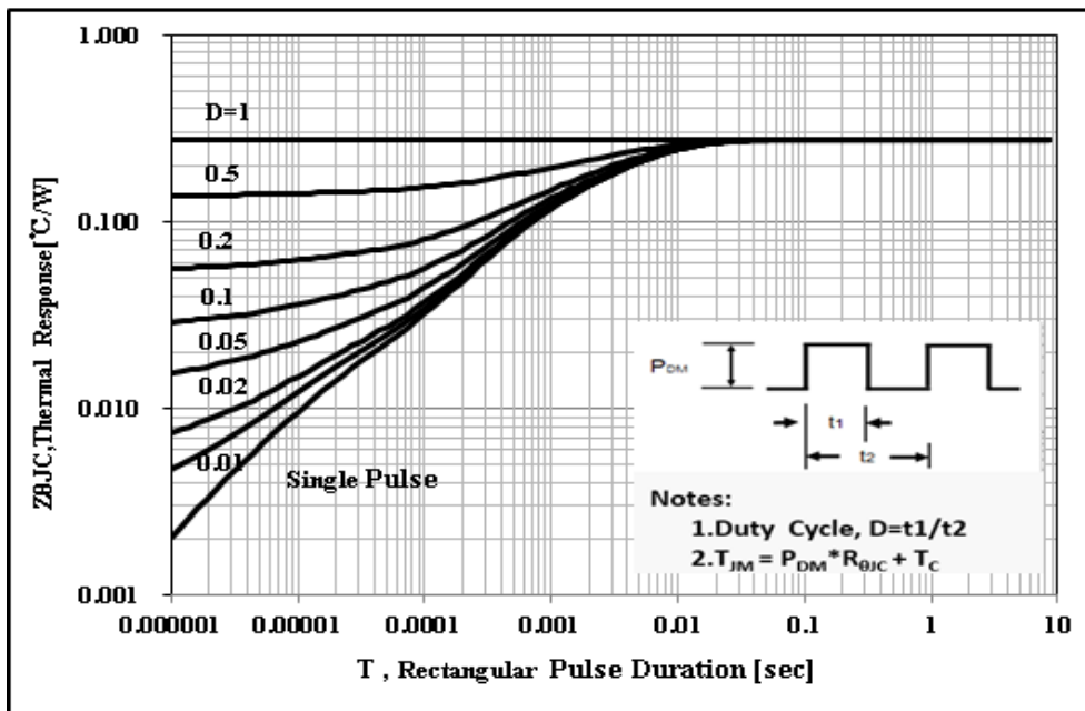
图 20 瞬态热阻特性
