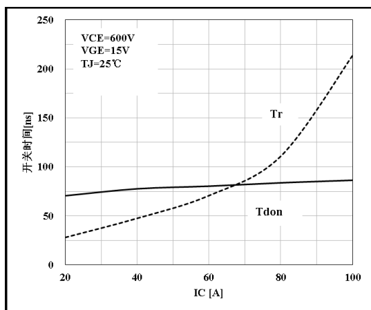
图 13 开通电流特性
