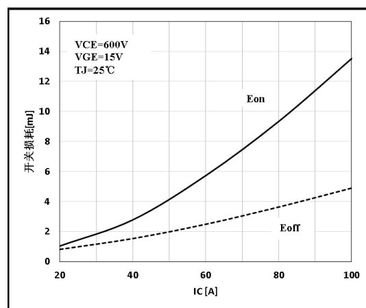
图 12 开关损耗电流特性
