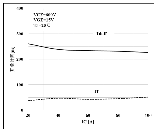
图 14 关断电流特性
