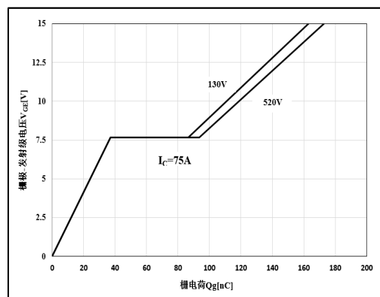
图 18 栅电荷特性
