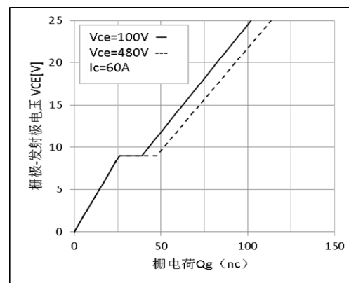
图 18 栅电荷特性
