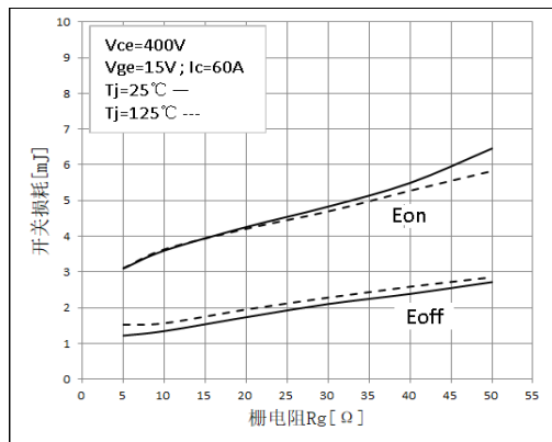
图 6 开关损耗-栅电阻特性曲线
