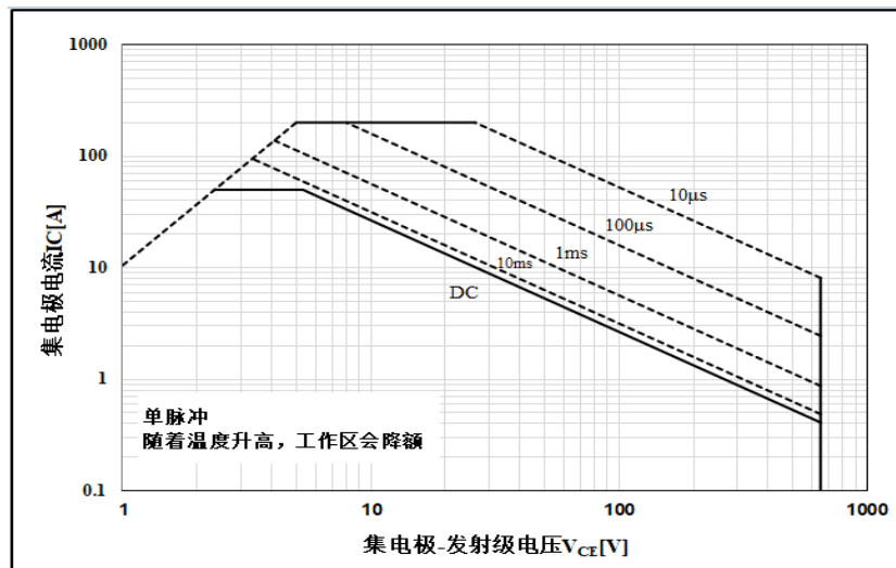
图 19 正向安全工作区
