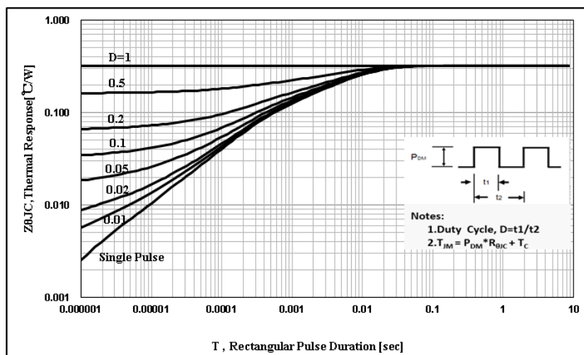
图 20 瞬态热阻特性
