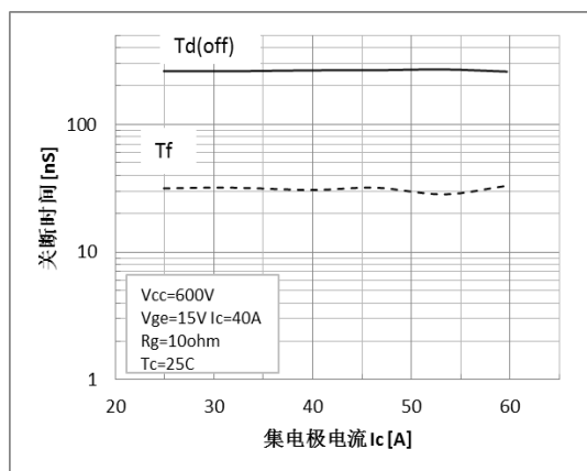
图 15 关断与电流特性
