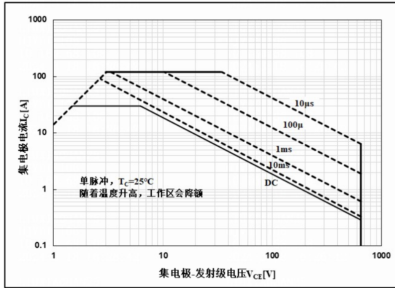
图 19 正向安全工作区
