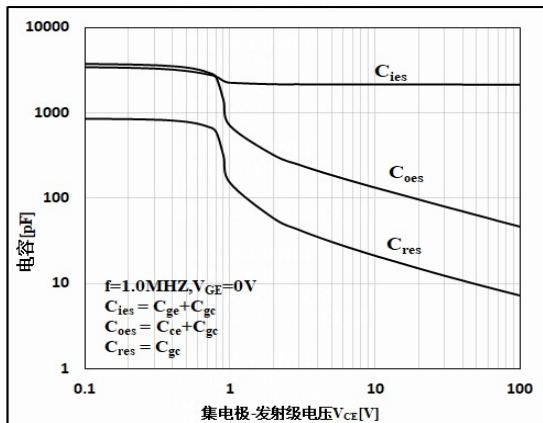
图 5 电容特性
