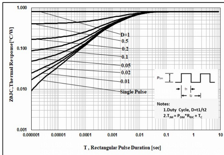
图 20 瞬态热阻特性
