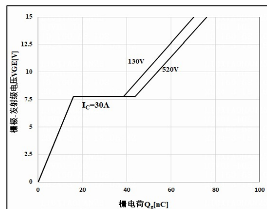
图 18 栅电荷特性
