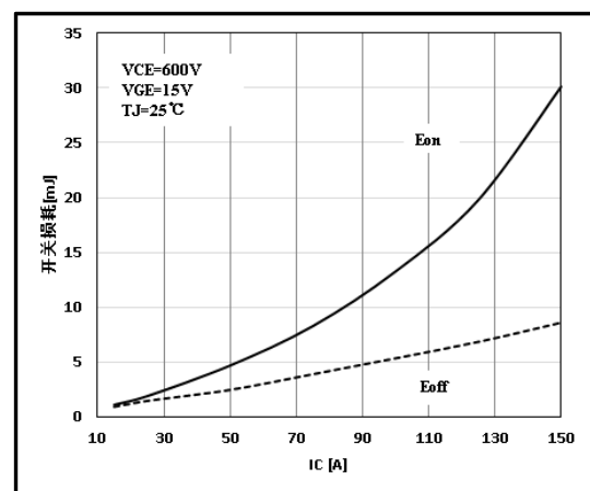
图 12 开关损耗电流特性
