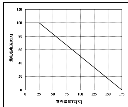
图 16 集电极电流温度特性 ( T_J \leq 175^\circ\text{C} )
