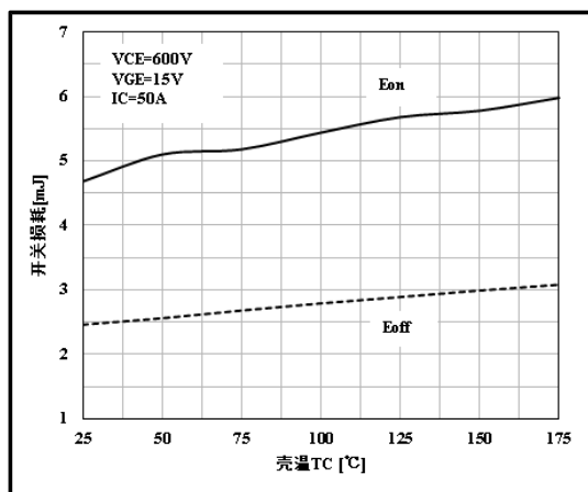
图 9 开关损耗温度特性
