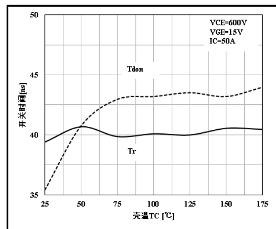
图 10 开通温度特性
