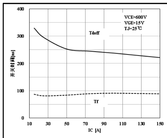
图 14 关断电流特性
