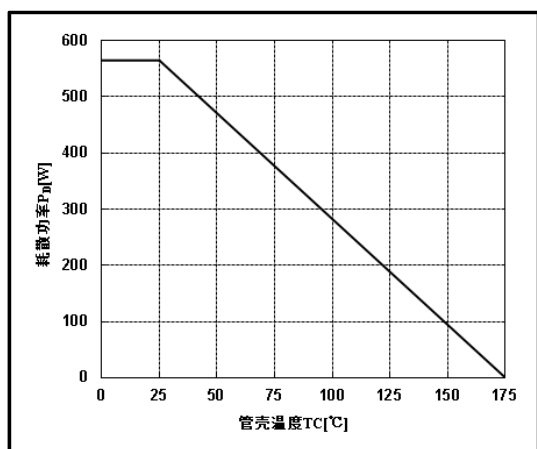
图 17 耗散功率温度特性 ( T_J \leq 175^\circ\text{C} )
