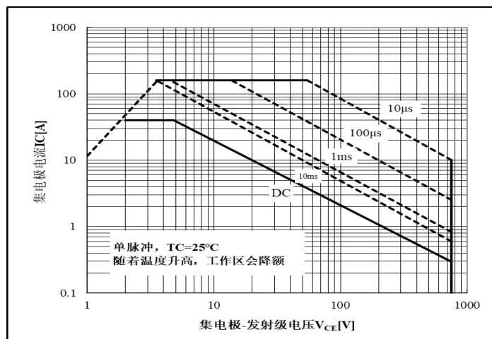
图 19 正向安全工作区
