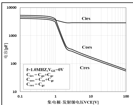
图 5 电容特性
