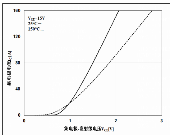
图 3 饱和和压降特性
