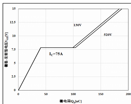
图 18 栅电荷特性
