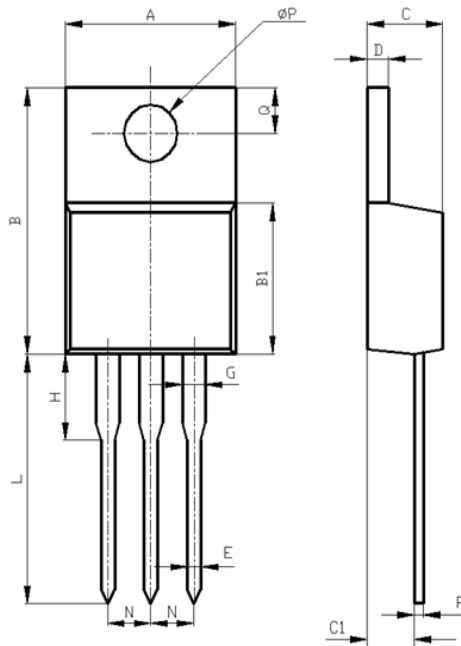
外形图：CRG15T65R85SDZ（TO-220）
