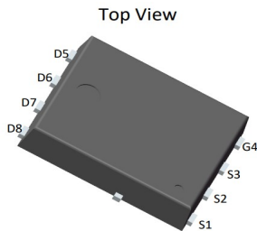
CRSM009N04L2
