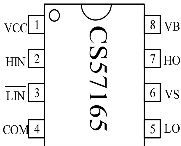
引脚排列图
